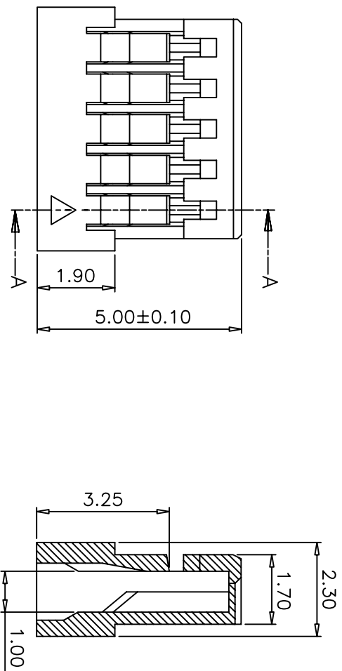
Section A-A
