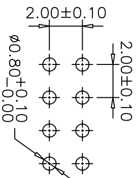
P.C.B LAYOUT
