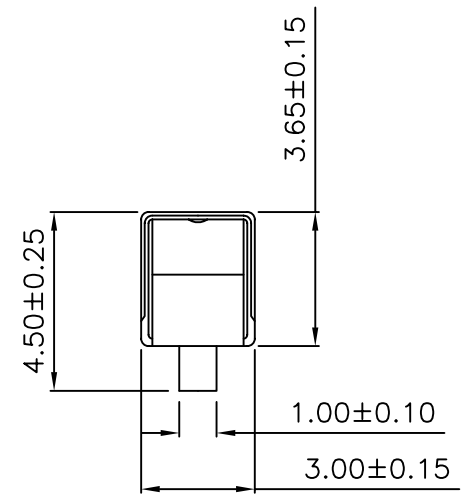
C-C
