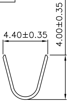
A-A
